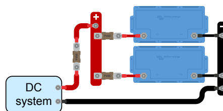
Più batterie in parallelo
