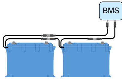
Połączenie BMS z dwoma akumulatorami (z opcjonalnymi kablami przedłużającymi)
