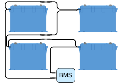
Połączenie BMS z kilkoma akumulatorami
