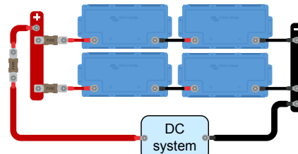
Mai multe baterii în serie/paralel
