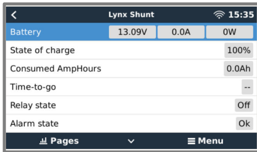
Appareil GX affichant les données opérationnelles du Lynx Shunt VE.Can
