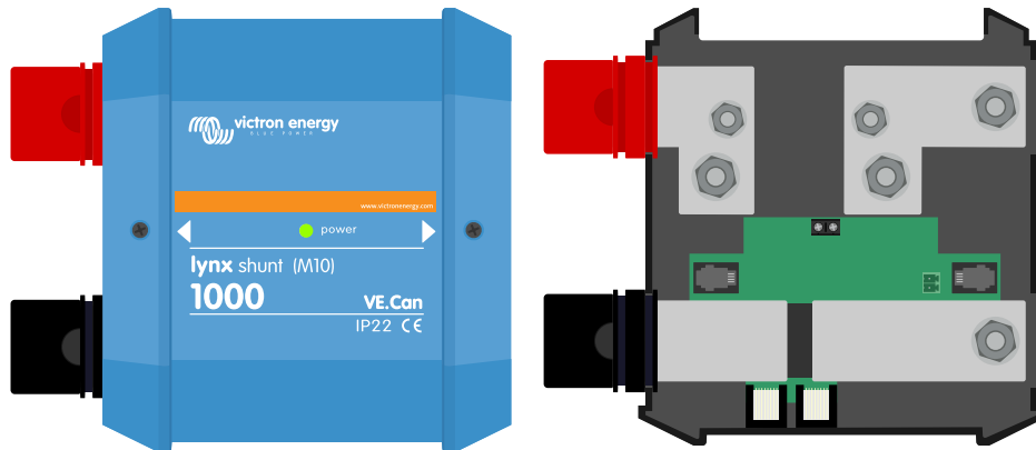
Der Lynx Shunt VE.Can (M8) – mit und ohne Schutzabdeckung
