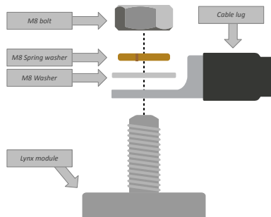
Figura 4. Secuencia de montaje correcta de los cables CC
