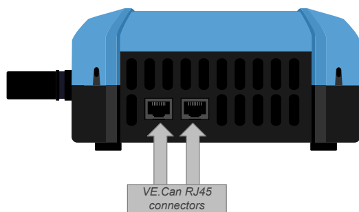
Ubicación de los conectores VE.Can del Lynx Shunt VE.Can
