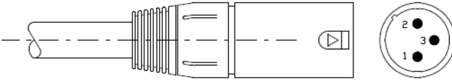
Figura 1 Connettore XLR
