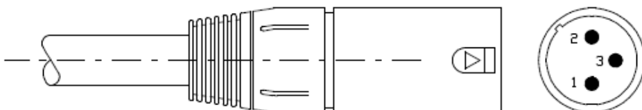
Figur 1 XLR-ladestik
