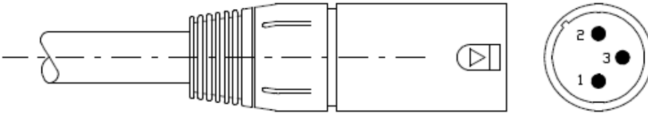
Obrázek 1 XLR-konektor
