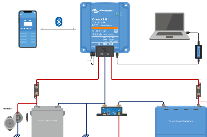
Typische Anschlüsseinstellung als DC-DC-Batterieladegerät
