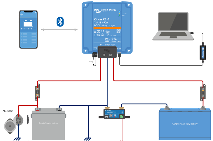
Kenmerkende aansluitingsinstelling als DC-DC acculader
